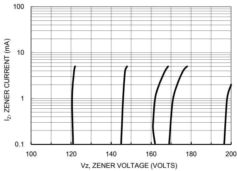
FIG. 8- V_z = 100 - 200 VOLTS
